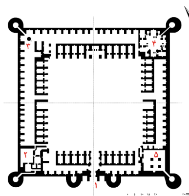
تصویر ۵: پلان کاروانسرای دیر گچین
