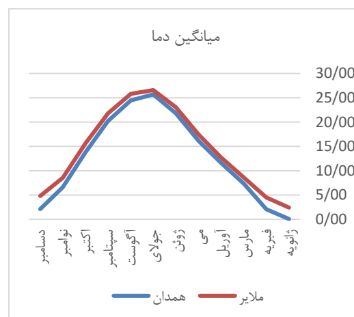
نمودار ۱: مقایسه میانگین دمای ماهیانه در همدان و ملایر
