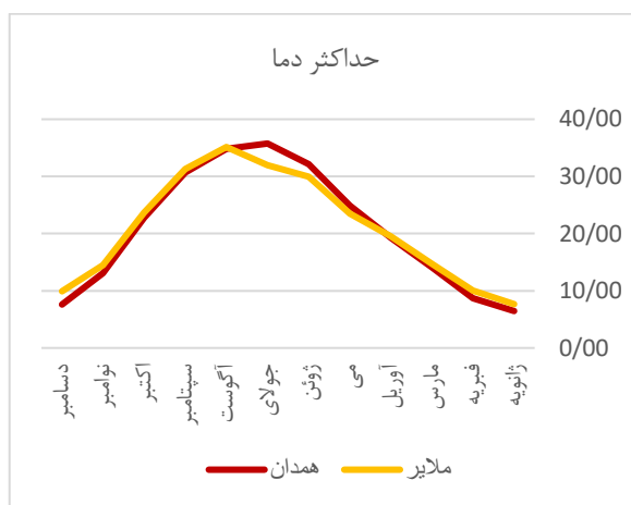
نمودار ۲: مقایسه حداکثر دمای ماهیانه همدان و ملایر
