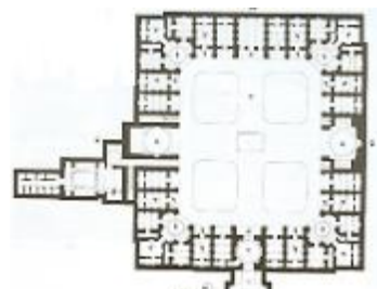
شکل ۴: از سمت راست به ترتیب پلان، ایزومتریک، شمای کلی مدرسه نیم آورد (ماخذ نگارندگان)
